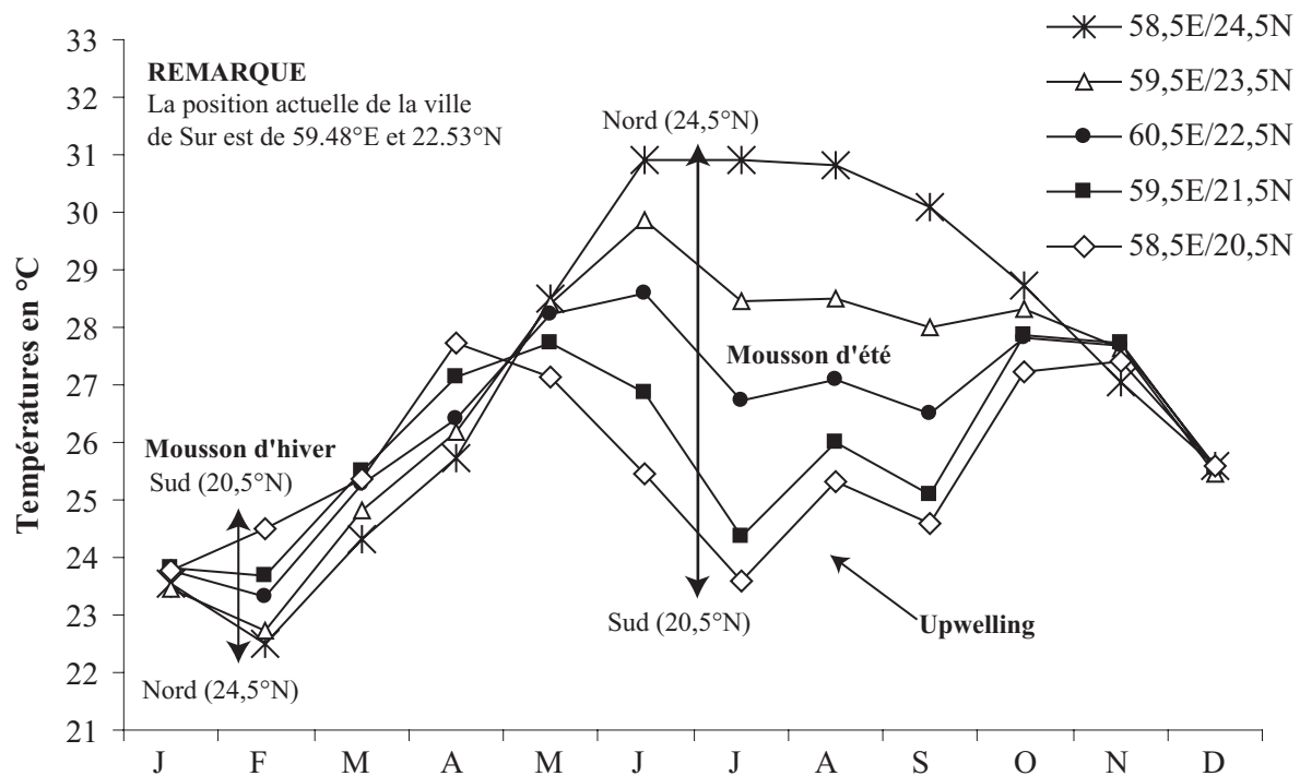
Figure 9 : Températures marines actuelles de surface en fonction de la position des sites du Nord au Sud du Ja'alan. Les upwellings sont visibles pour les sites au Sud (20,5°N). (Levitus, 1982)
