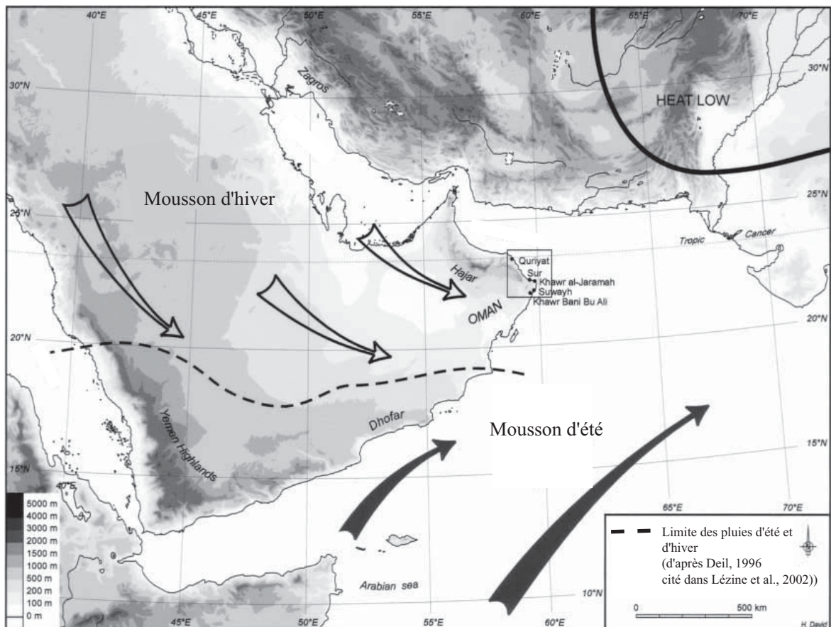
Figure 4 : Limites actuelles des pluies de moussons d'hiver et d'été sur la péninsule Arabique (d'après Lézine et al., 2002)
