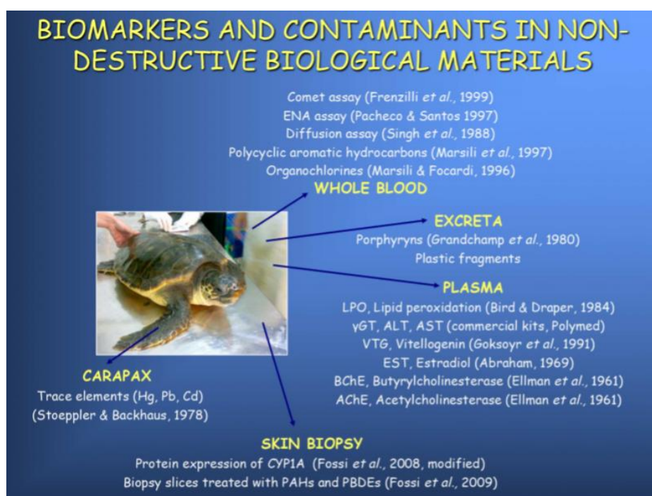
Figure 1. Méthodes et biomarqueurs utilisés, et contaminants recherchés chez la tortue Caouanne, par l'Université de Sienne (Italie) par type d'échantillon. Les références des travaux décrivant la méthode d'analyse utilisée figurent entre parenthèses. D'après Casini, 2015.
