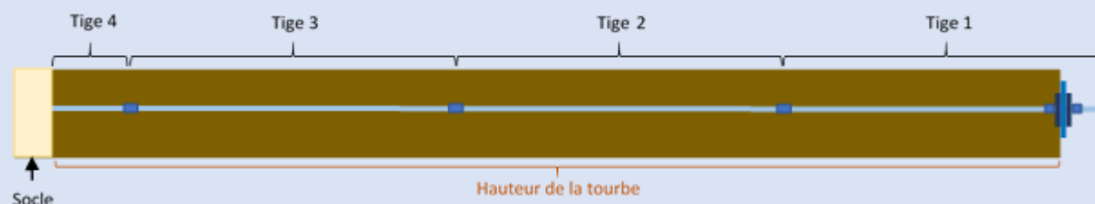
Figure 3 : Schéma de l'installation d'une perche constituée de plusieurs tiges fixées bout-à-bout de la surface jusqu'au socle
