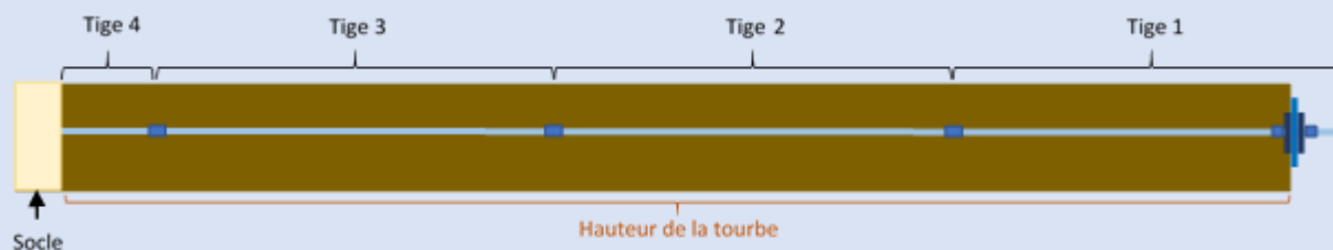
Figure 3 : Schéma de l'installation d'une perche constituée de plusieurs tiges fixées bout-à-bout de la surface jusqu'au socle
