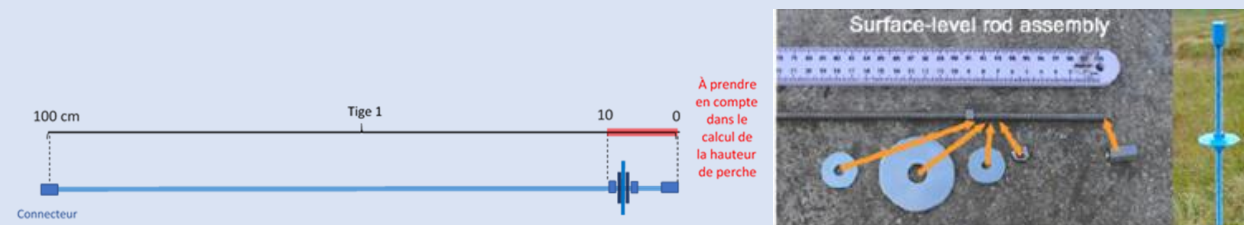
Figure 2 : Explicatif d'un montage de tige (Lindsay et al., 2019)
