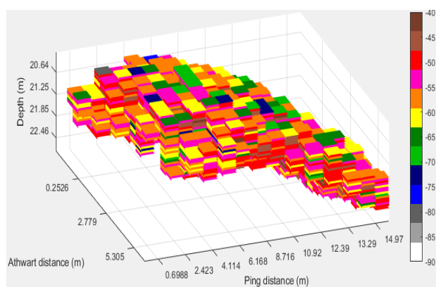
Figure 12. Observation 3-D d'un banc enregistré par le sonar multi-faisceaux. Les couleurs représentent les différents niveaux d'intensité acoustique (en dB).
