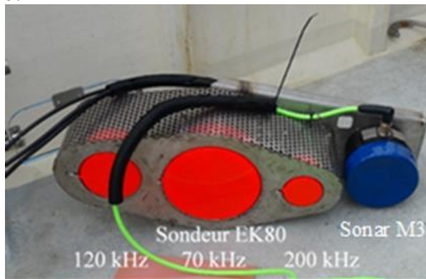
Figure 10. Photographie du matériel acoustique avec en orange à gauche les 3 fréquences de l'EK80 et en bleu à droite le M3 (a). Représentation schématisée des deux systèmes acoustiques, le sonar multifaisceaux M3 (gris clair) avec sa fauchée large ( 120^\circ ) et le sondeur split-beam EK80 (gris foncé) avec sa faible fauchée ( 7^\circ ) (b).
