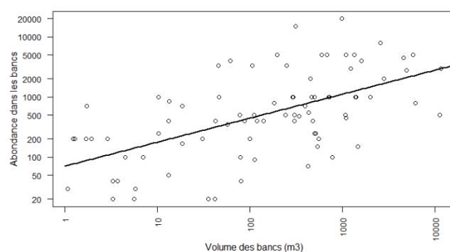
Figure 24. Relation entre l'abondance de poissons pélagiques dans les bancs observés par les plongeurs et le volume des bancs (m³) obtenu avec le sonar M3 après extraction sous Matecho
