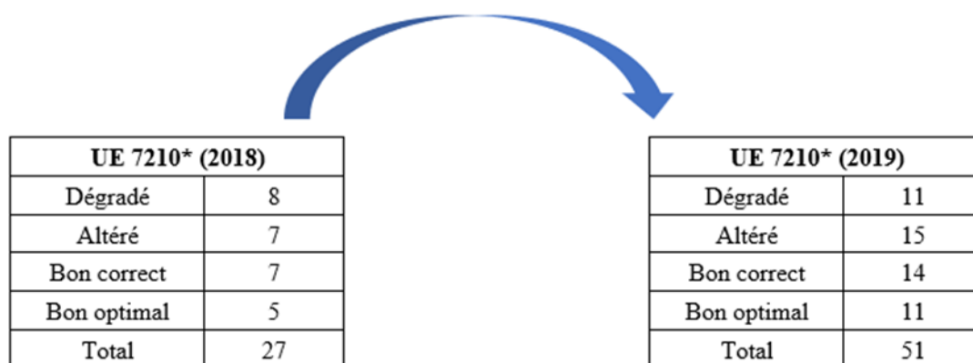
Figure 28. Nombre de relevés effectués en 2018, puis en 2019, sur les cladiaies.
