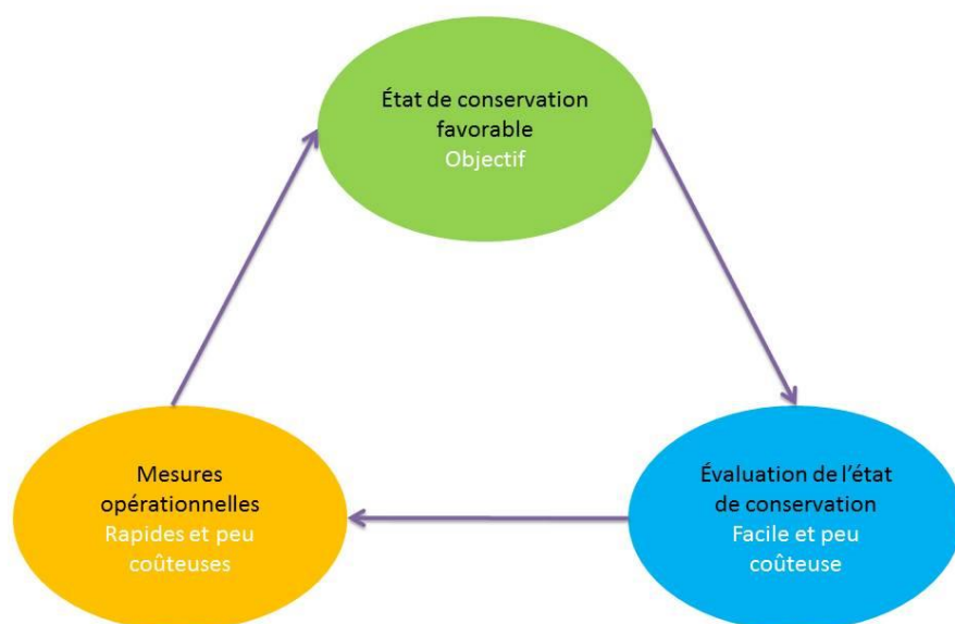
Figure 16. Processus cyclique mettant en avant la démarche scientifique (en noir) et les ambitions opérationnelles (en blanc) dans la mise en œuvre de la DHFF.
