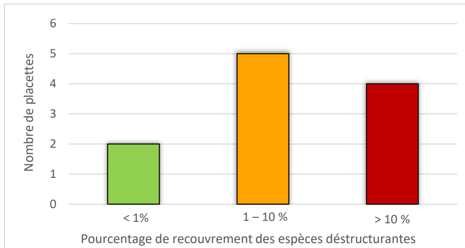
Figure 14. Nombre de placettes échantillonnées au sein d'un site Natura 2000 selon les résultats de l'indicateur « Recouvrement des espèces destructurantes ».
