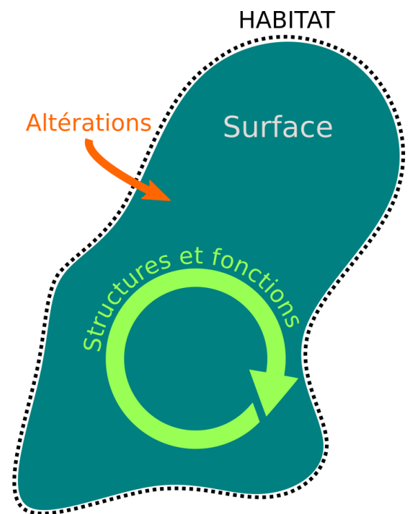
Figure 6. Schéma des trois paramètres pris en compte dans l'évaluation de l'état de conservation de l'habitat à l'échelle des sites Natura 2000.
