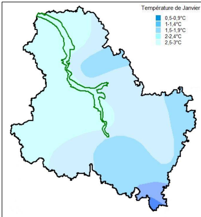
Fig. 3 : Températures moyennes de Janvier (in Bardet et al 2008)
