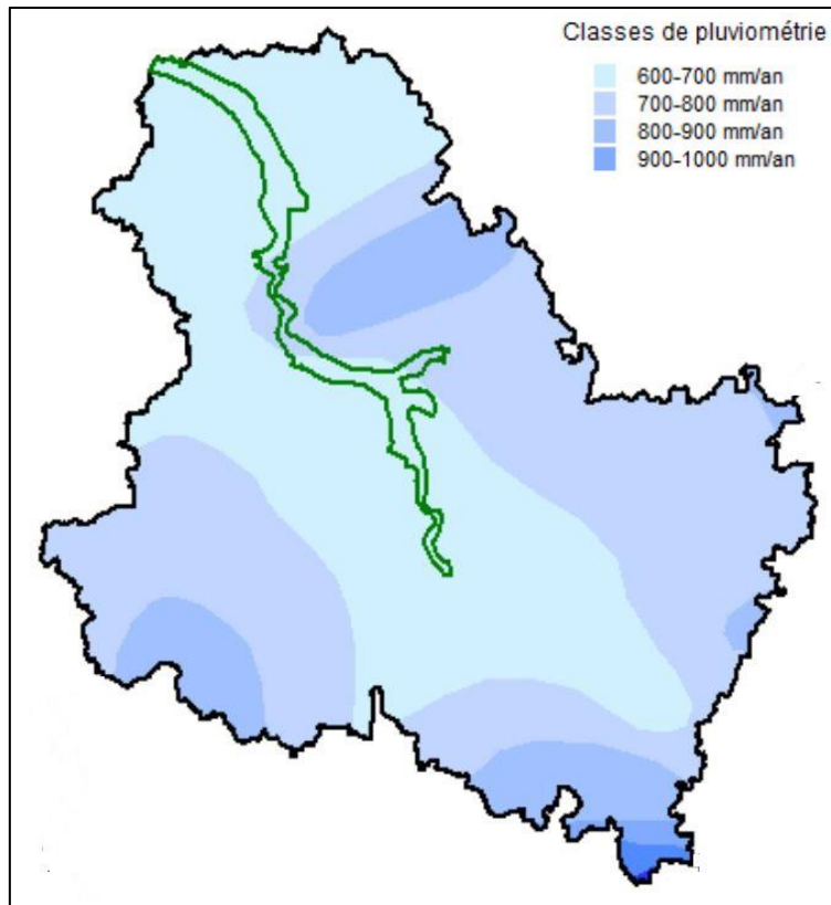
Fig. 5 : Classes de pluviométrie (in Bardet et al 2008)
