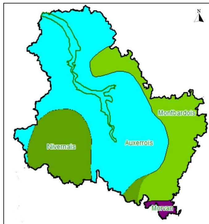
Fig. 2 : Régions climatiques (in Bardet et al 2008)
